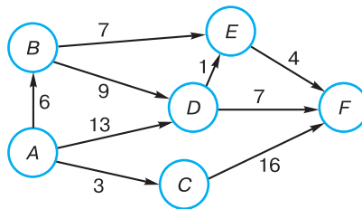
Рис. 3.7. Ориентированный граф
