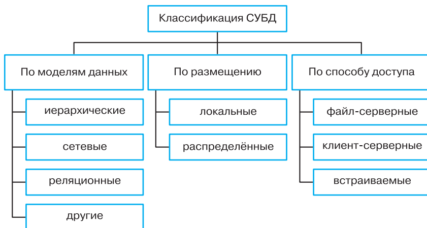
Рис. 3.31. Классификация СУБД
