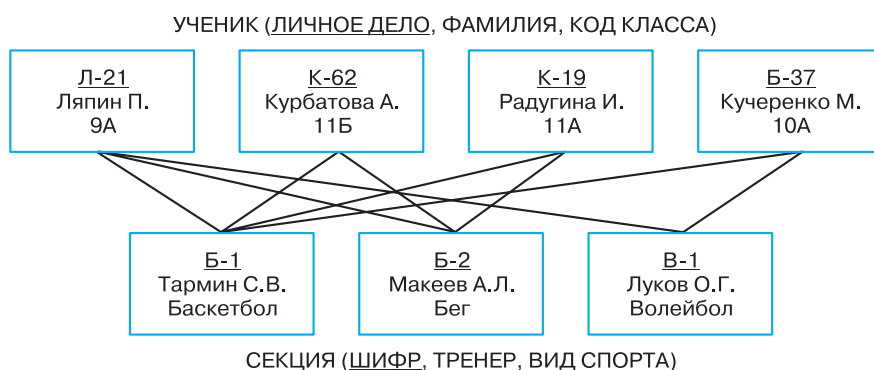
Рис. 3.25. Сетевая структура данных
