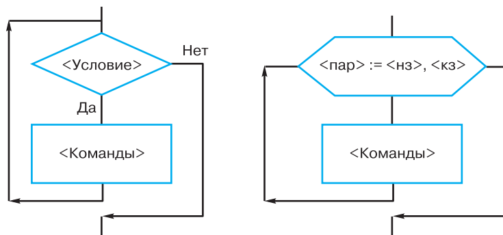
Рис. 2.8. Блок-схемы циклов
